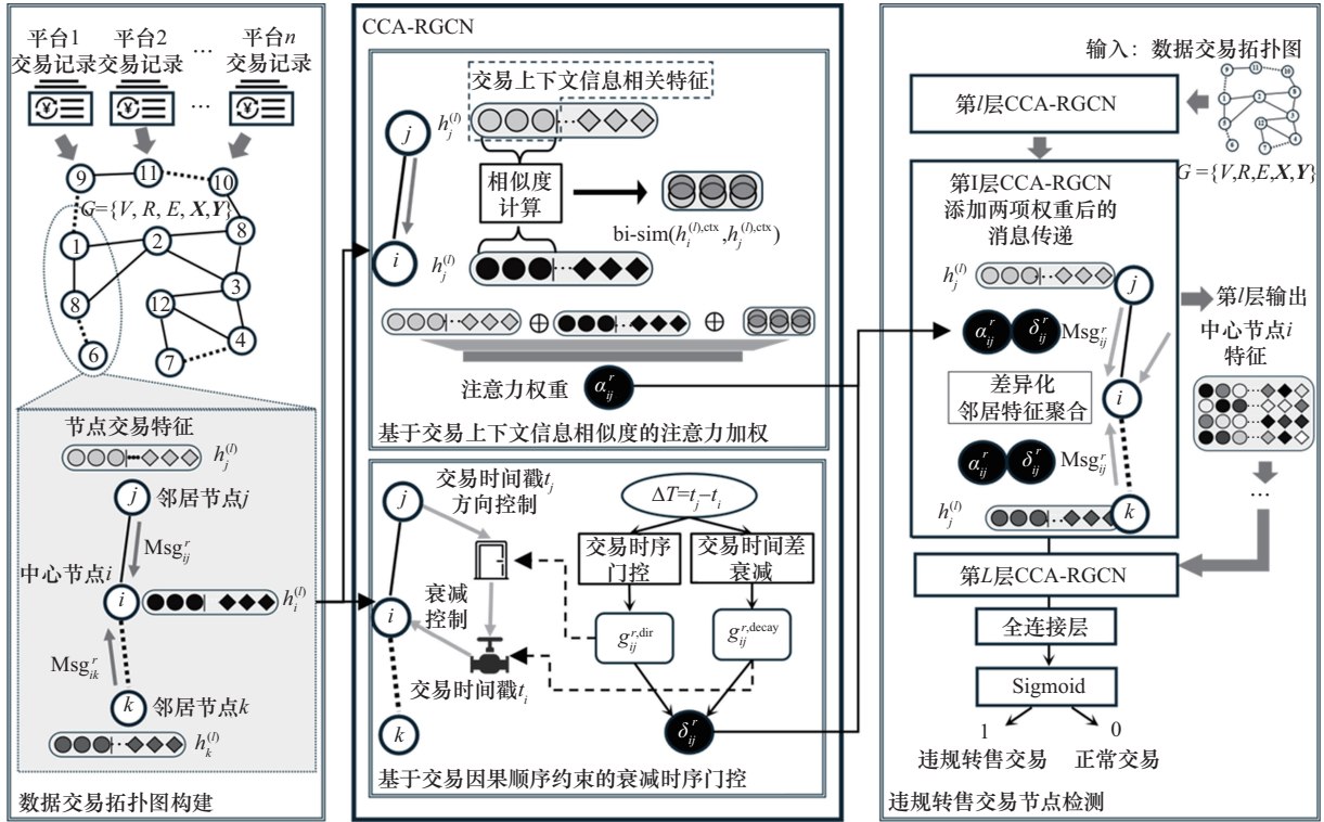
图2 基于CCA-RGCN的数据违规转售检测方法架构
